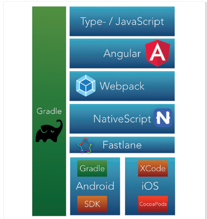
Abbildung 2: Technologie-Stack
